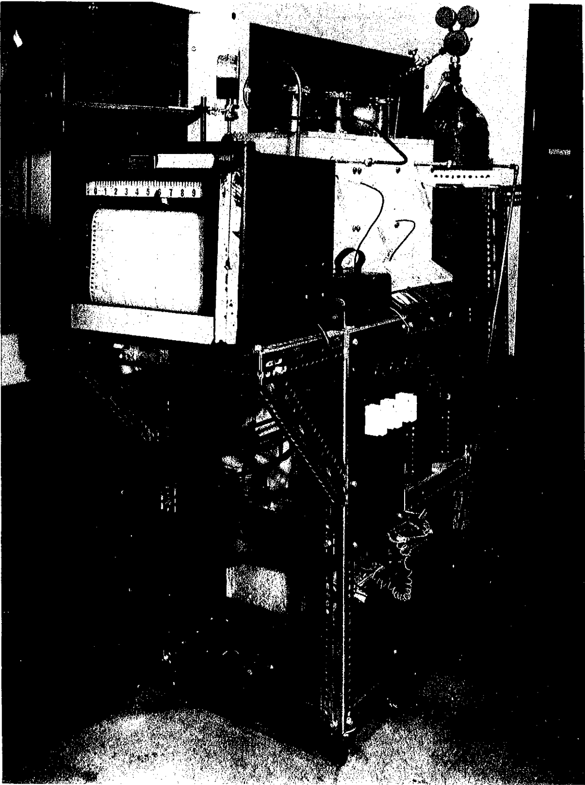
Fig. 8a. Argon purification unit.
