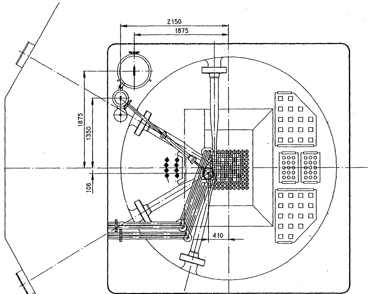
REACTEUR SIRIUS 2 PISCINE REACTEUR - VUE DE DESSUS VARIANTE AVEC SOURCE FROIDE
