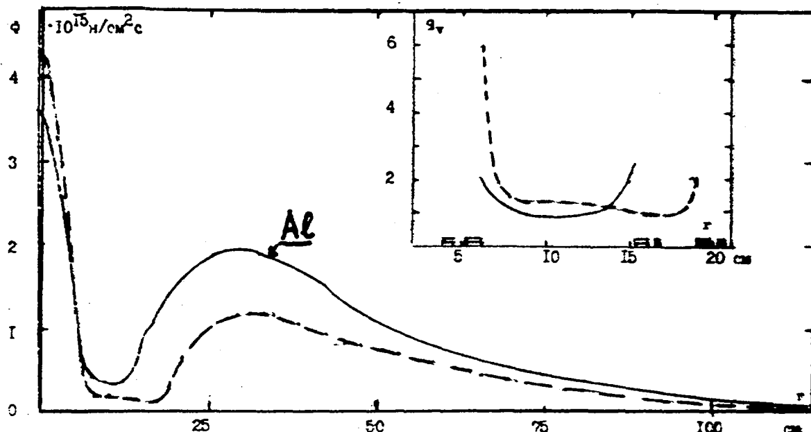
Рис.6. Распределение потока тепловых нейтронов \Phi и неравномерности энергоснабжения q_v по радиусу r в средней плоскости реактора при мощности 100 МВт. Сплошные кривые для водо-алюминиевой активной зоны ( w_{\text{акт}} = 0,413 ) с содержанием топлива 240 г ^{235}\text{U}/\text{л} , высотой 80 см и внешним радиусом 15 см. Пунктирные кривые для штатной конструкции активной зоны реактора ПИК. В обоих случаях в центре реактора размещена цилиндрическая легководная ловушка с алюминиевой направляющей.
